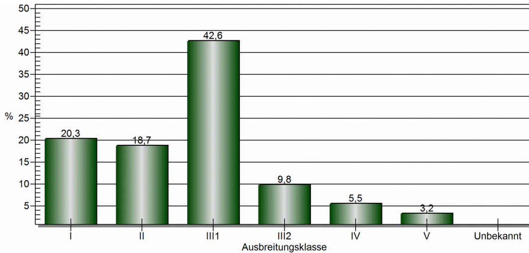
Bild 5.3. Häufigkeitsverteilung der Ausbreitungsklassen an der LANUV-Station Lünen-Niederaden des Jahres 2009 [11]
