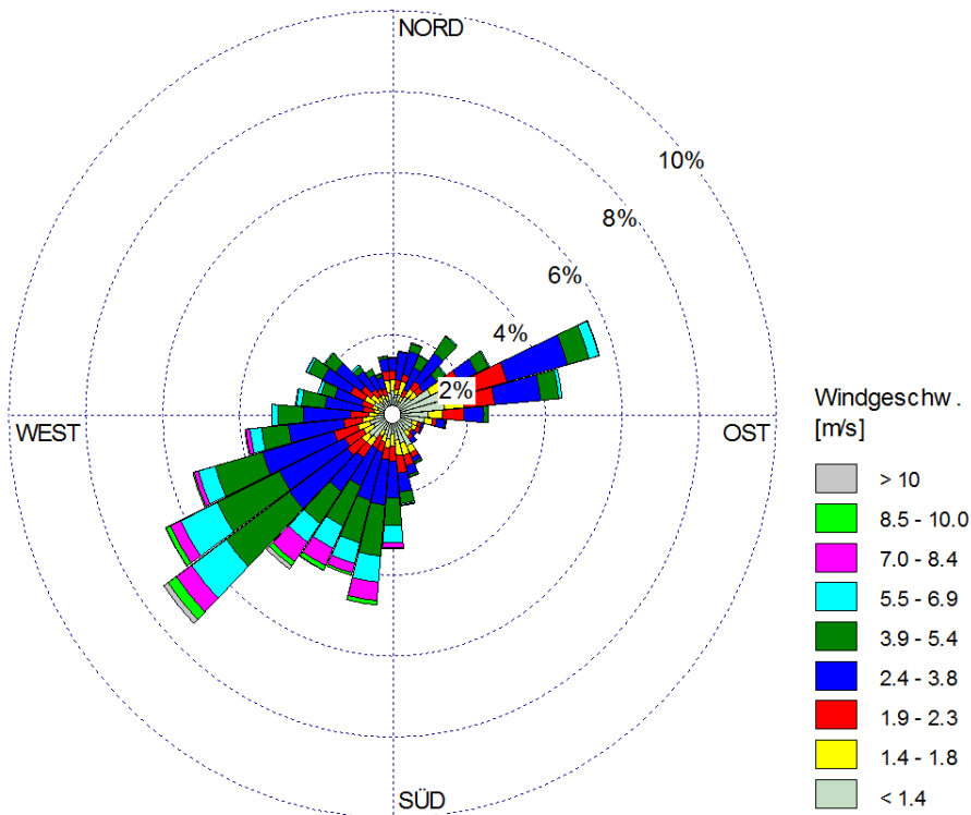
Bild 5.1. Häufigkeitsverteilung der Windrichtungen und Windgeschwindigkeiten an der LANUV-Station Lünen-Niederaden des Jahres 2009 [11]
